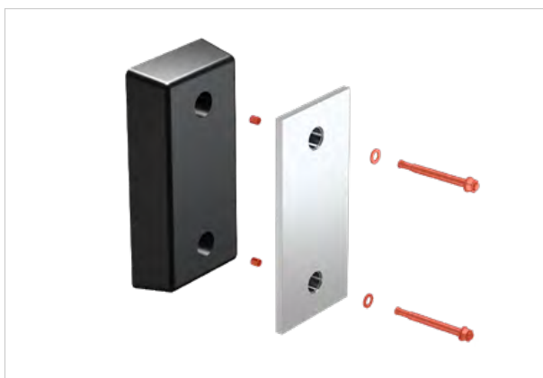
Комплект крепления пластины монтажной к бетону МРМ
